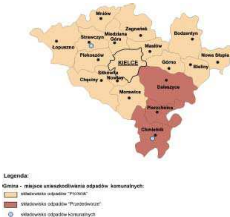
Rys. 8.1.1e. Miejsca unieszkodliwiania odpadów komunalnych w rejonie centralnym do końca 2009 r.
