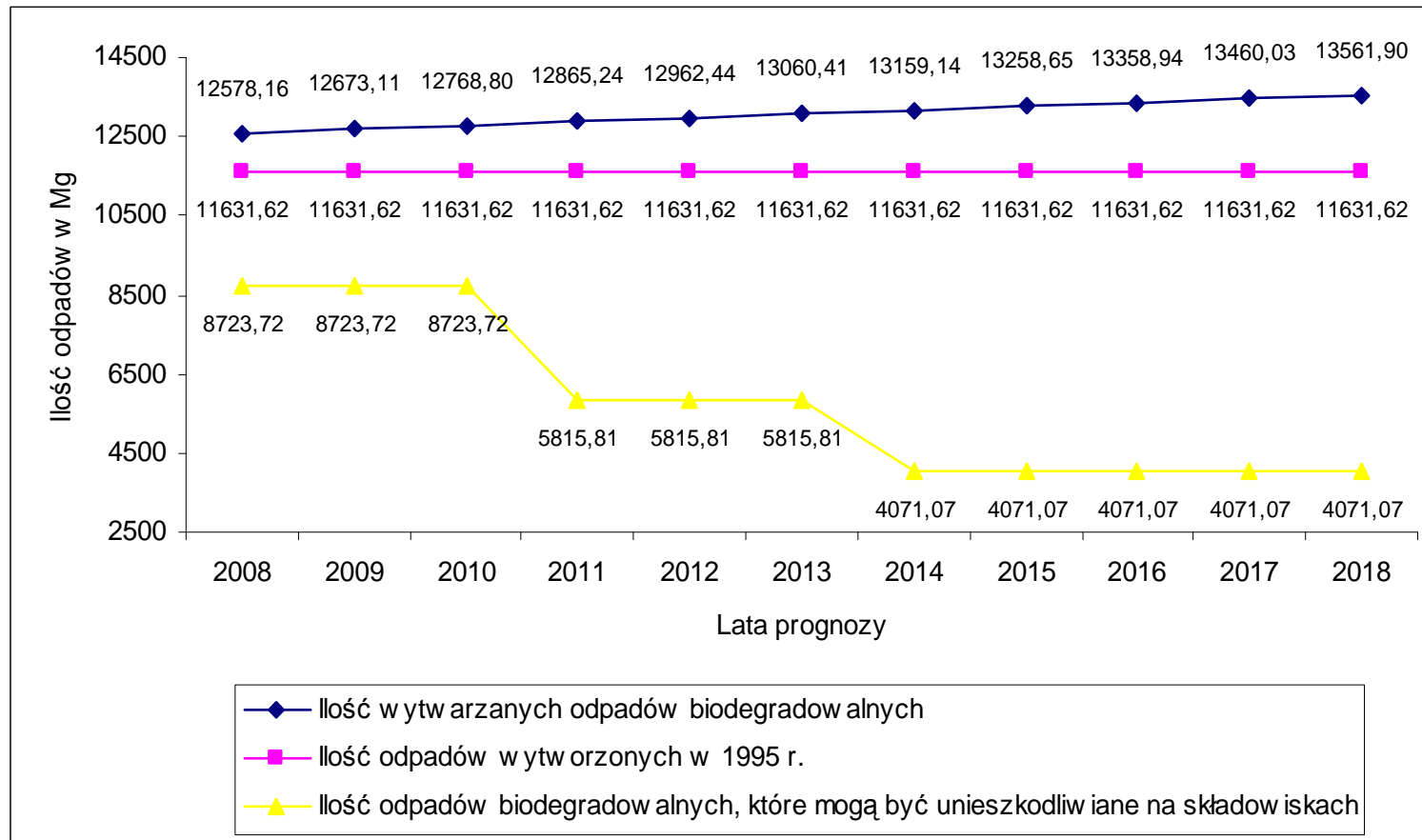
Rys. 5.1b. Prognoza ilości wytwarzanych odpadów ulegających biodegradacji oraz ilości dopuszczalnych do składowania, w Mg
