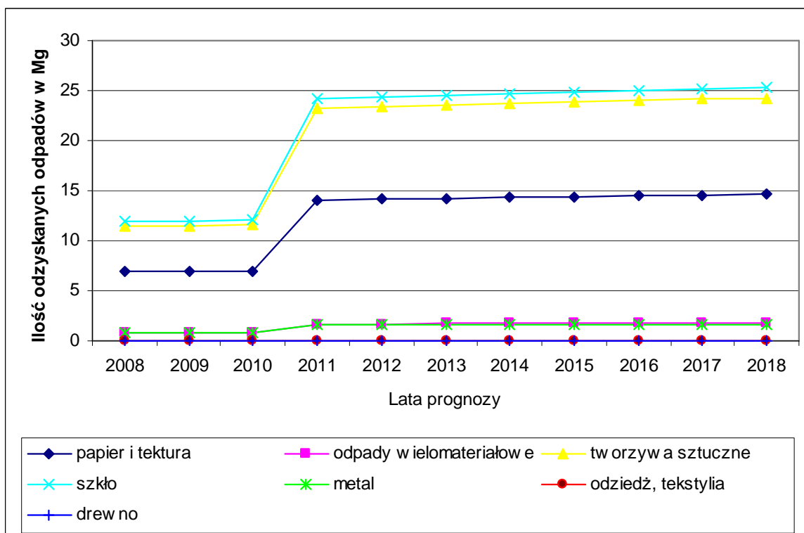
Rys. 5.2.10d. Prognoza odzyskania odpadów opakowaniowych na terenie Gminy Raków, w Mg
