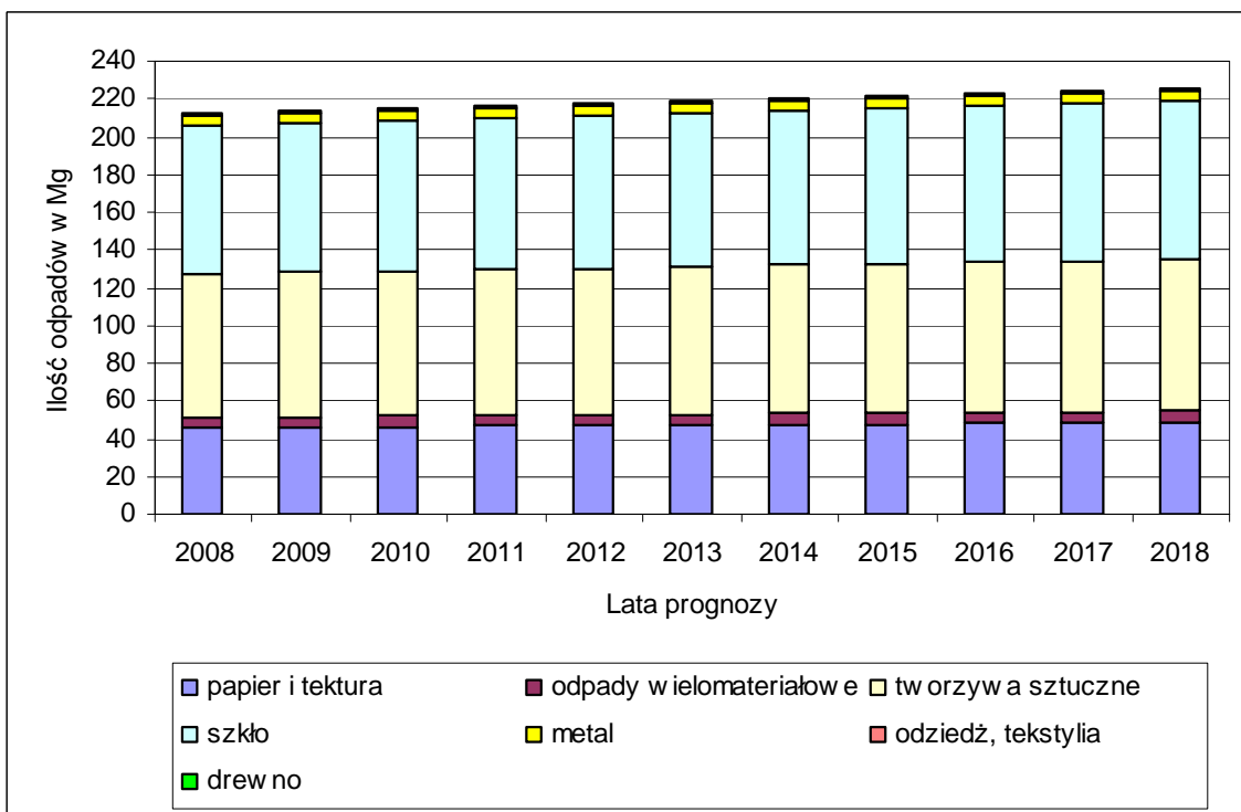
Rys. 5.2.2c. Prognoza ilości i rodzaje odpadów opakowaniowych wytwarzanych na terenie Gminy Pacanów, w Mg
