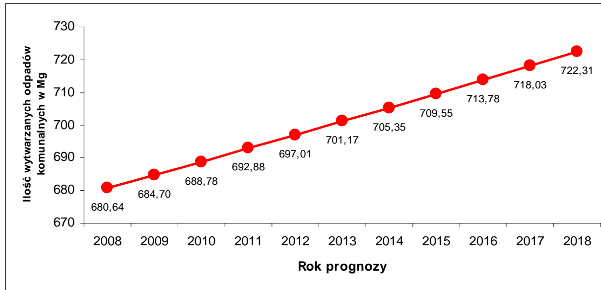
Rys. 5.2.15a. Prognoza wytwarzania odpadów komunalnych na terenie Gminy Łubnice, w Mg
